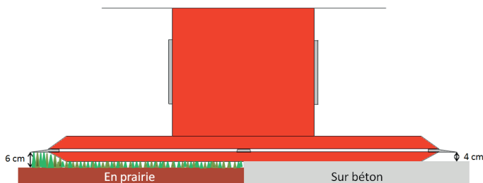
Abbildung 2. Einstellung der Messer eines Trommelmähers auf Grünland und auf Beton
